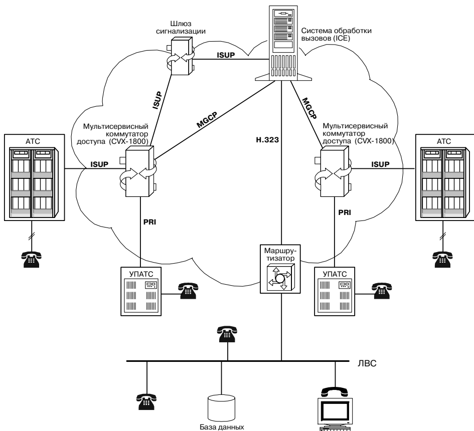
Рис. 8.7 Инфраструктура IPConnect
