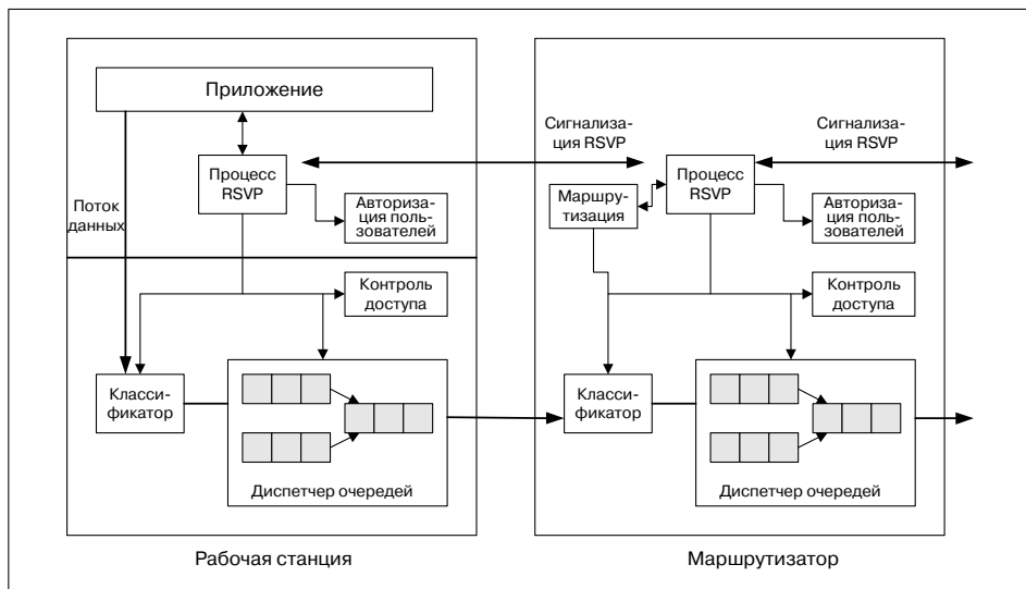
Рис. 10.2 Модель IntServ
